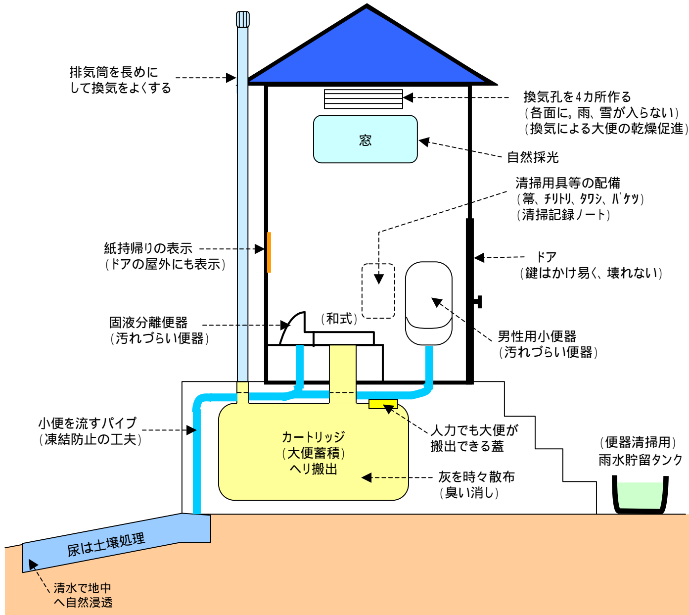
固液分離・尿貯留へり搬出・尿土壌処理方式
